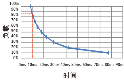
DDR-120B-24
