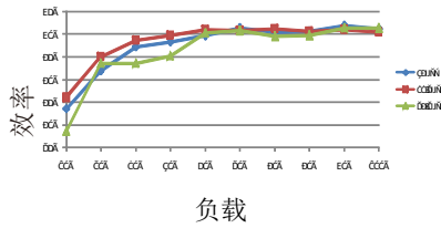
DDR-120C-24
