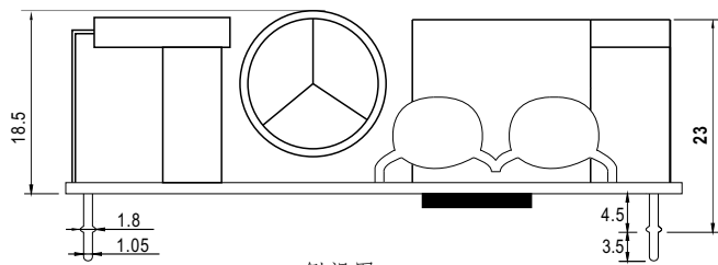
侧视图
